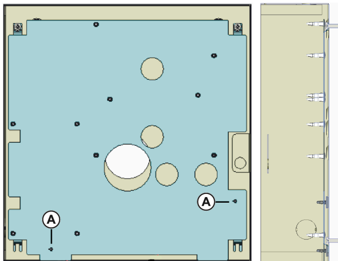
Illustration 2 : Installation de la plaque métallique dans un KT-300 (D31000201 rev 0/1)
